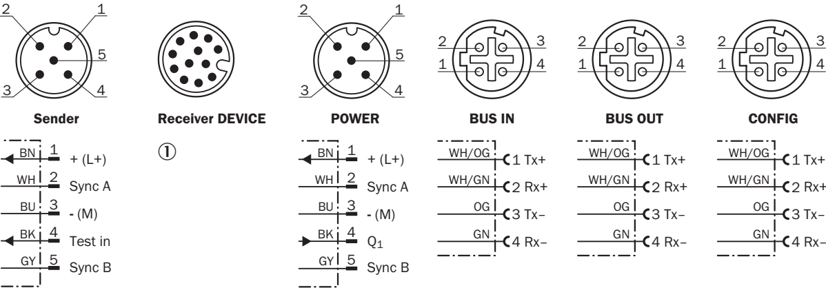
連接類型與接線圖 MLG-2 WEBCHECKER
