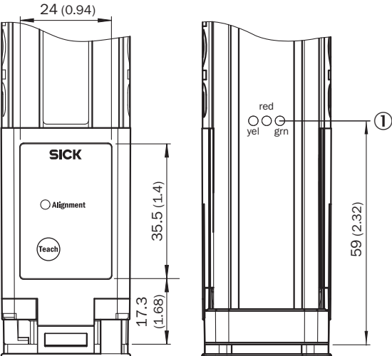
① statusindikering: LED:er grönn, gul, röd
