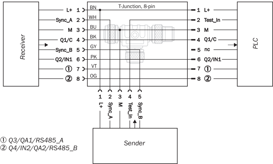
連接示意圖 T型接頭，可編程邏輯控制器
