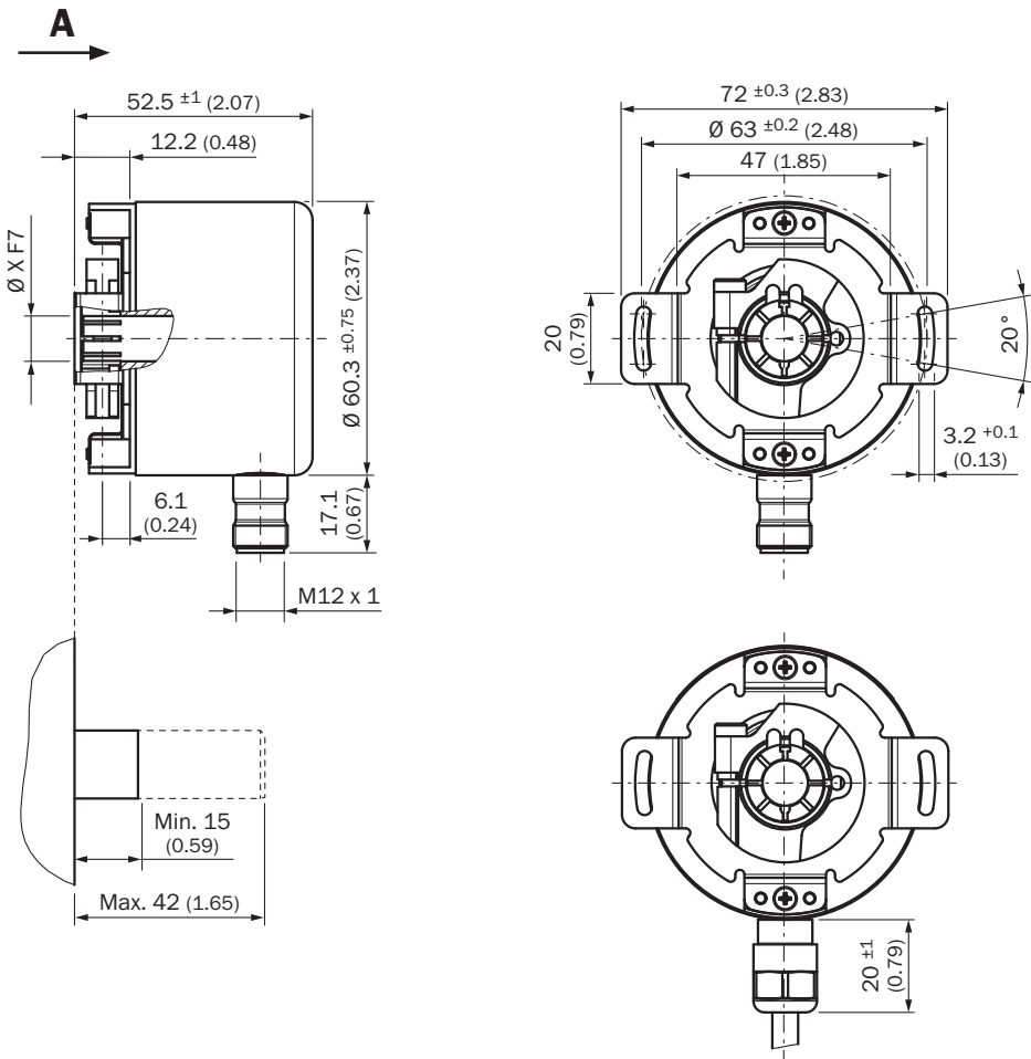
尺寸 (mm)
