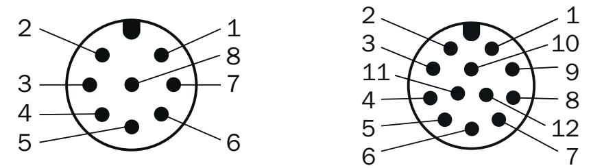
編碼器上M12公接頭視圖
