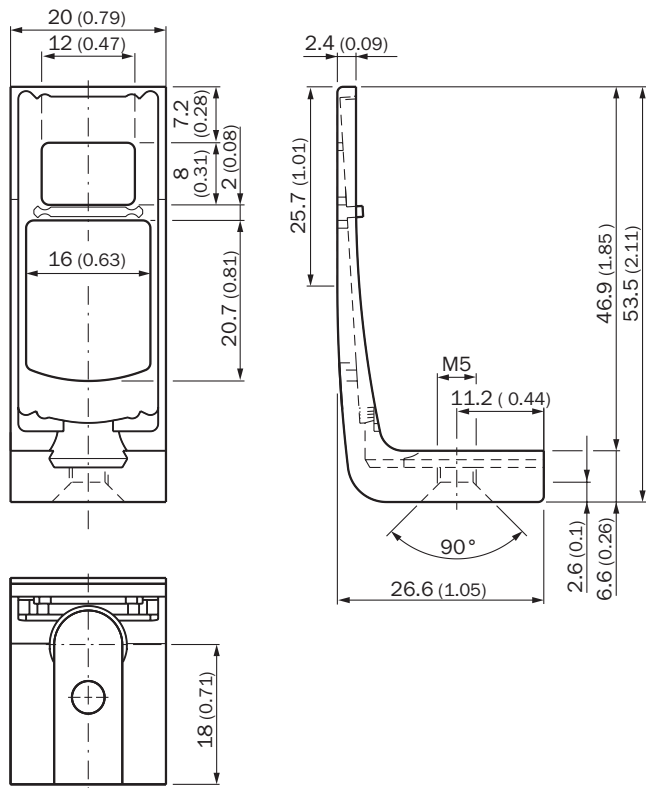
Размеры, мм
