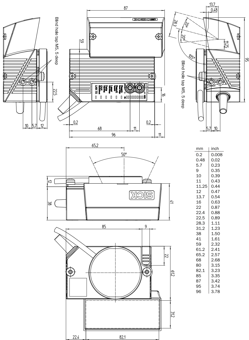
Размеры, мм
