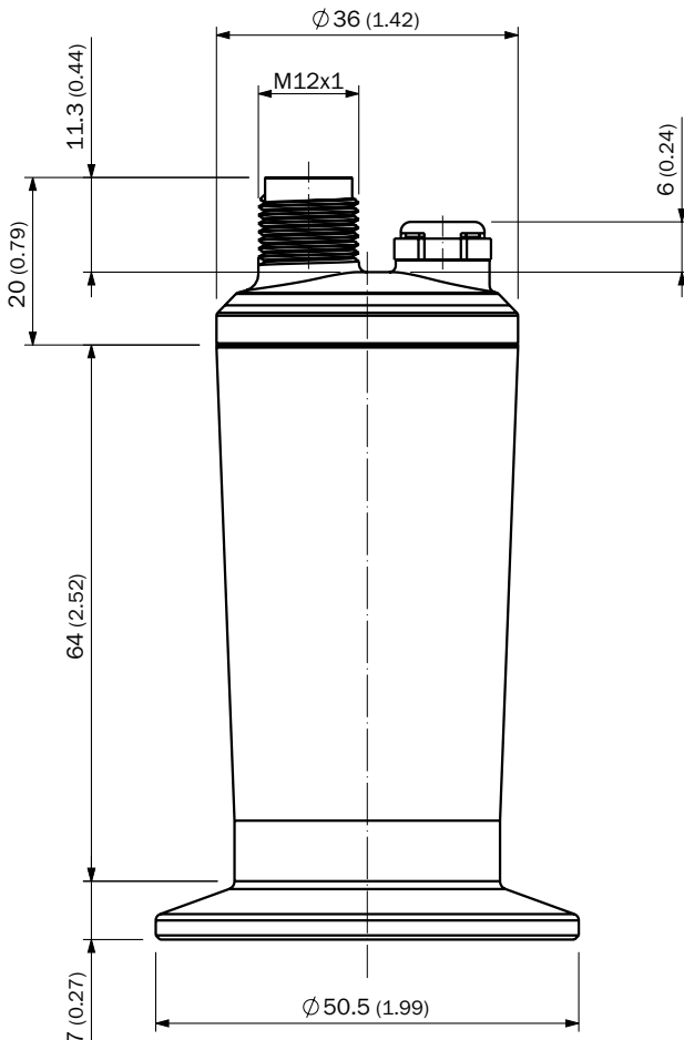
Размеры, мм
