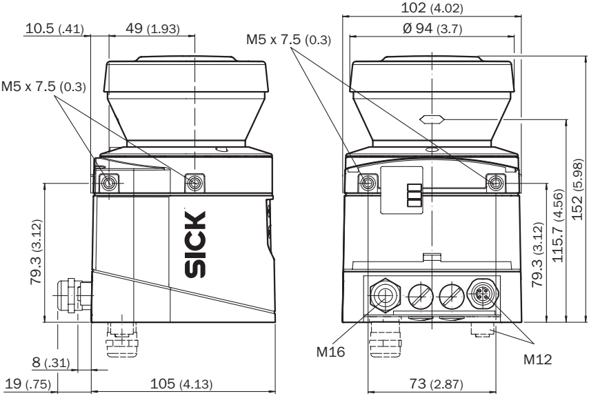
Размеры, мм
