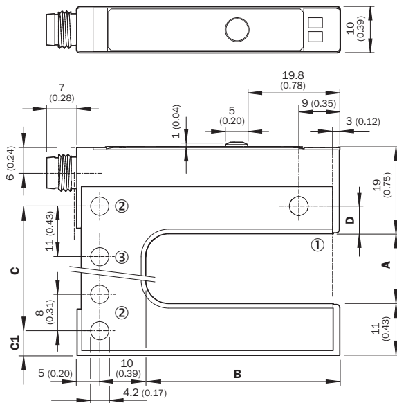
Размеры, мм
