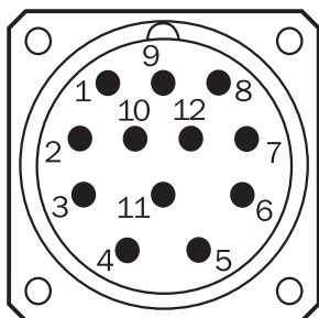
Вид приборного штекера M23 на энкодере
