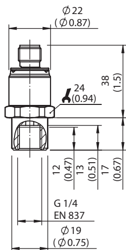
Размеры, мм
