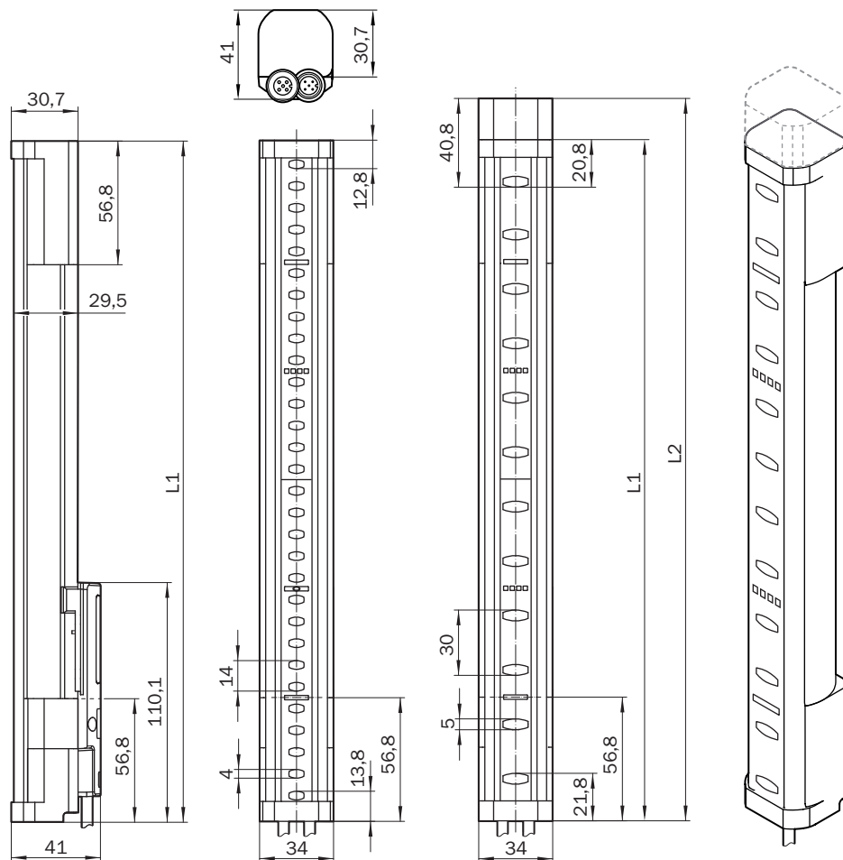
Размеры, мм
