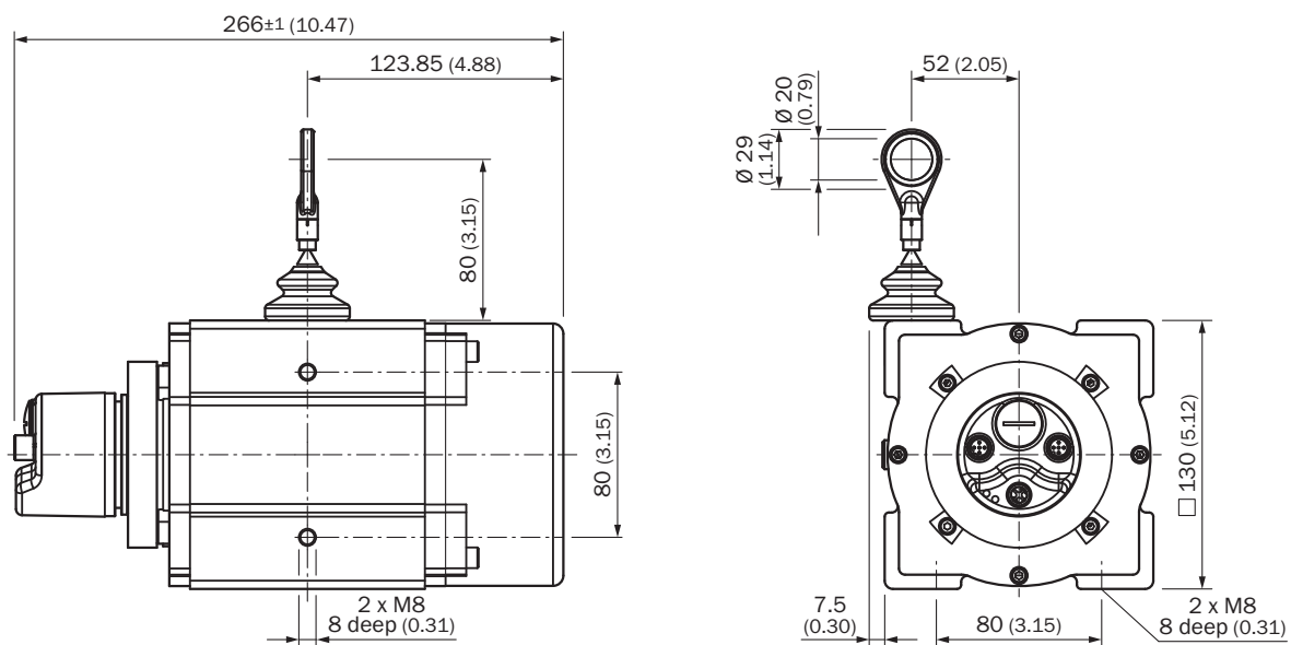
Размеры, мм
