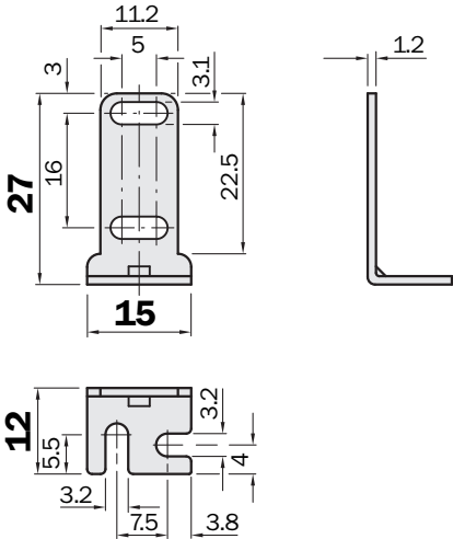
Размеры, мм
