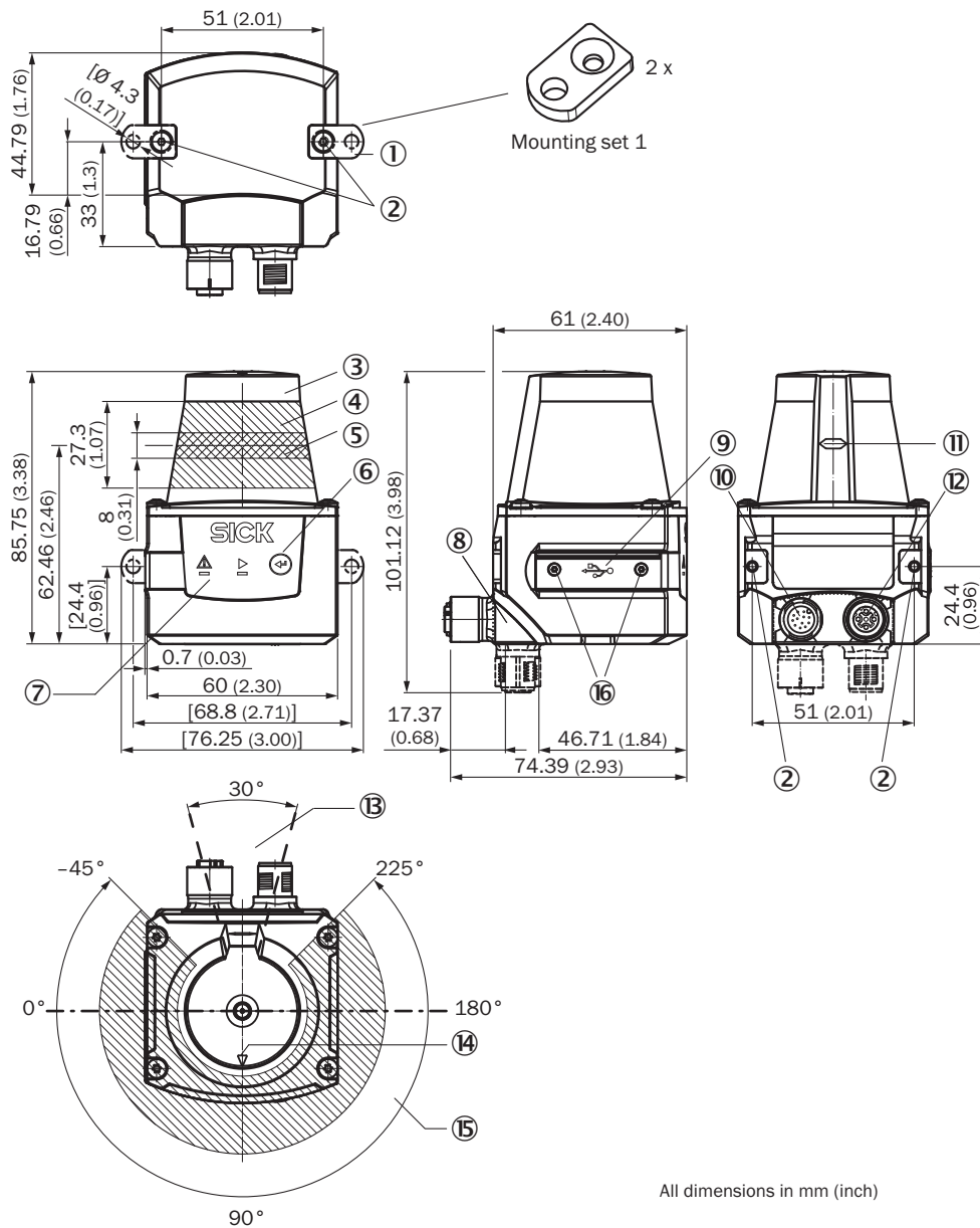
尺寸圖
