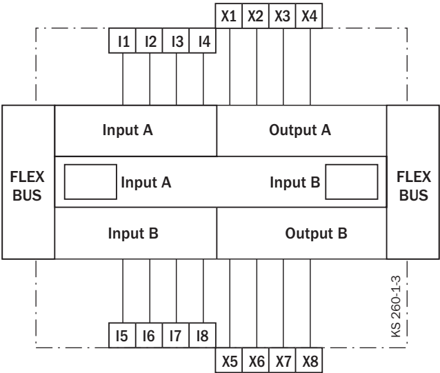
連接示意圖
