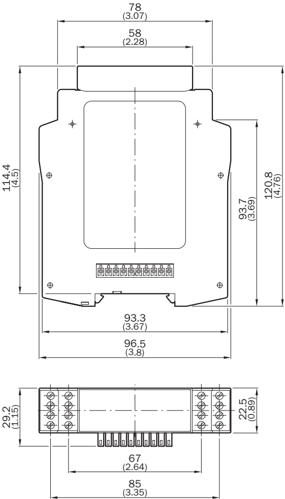
尺寸 (mm)
