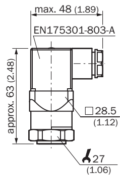
Размеры, мм
