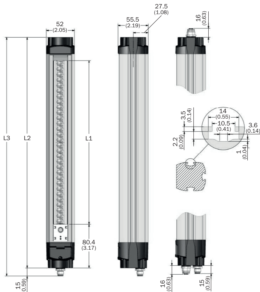
Размеры, мм
