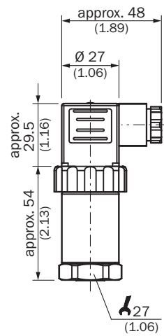
Размеры, мм
