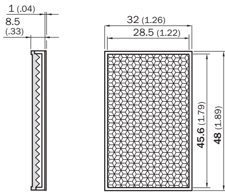
Размеры, мм
