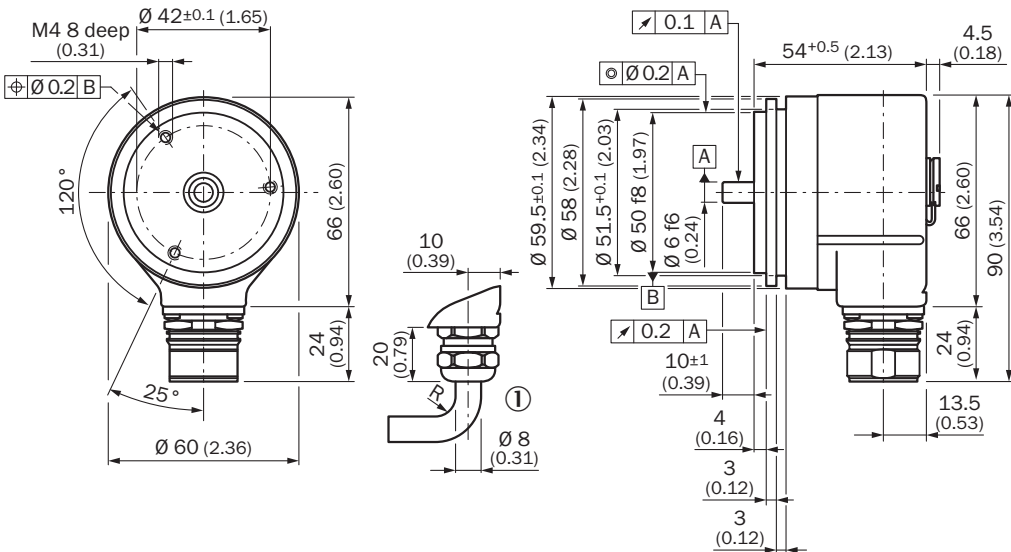
Габаритный чертеж (Размеры, мм)
