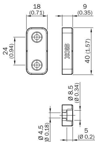
Размеры, мм
