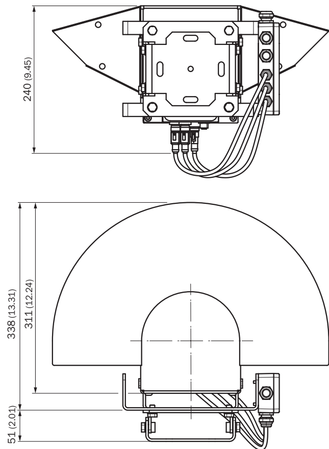
Размеры, мм Погодозащитный кожух 190°
