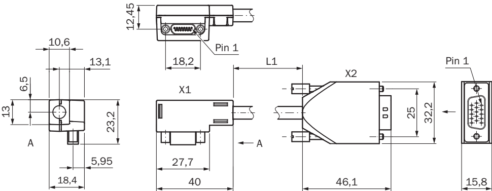
Размеры, мм
