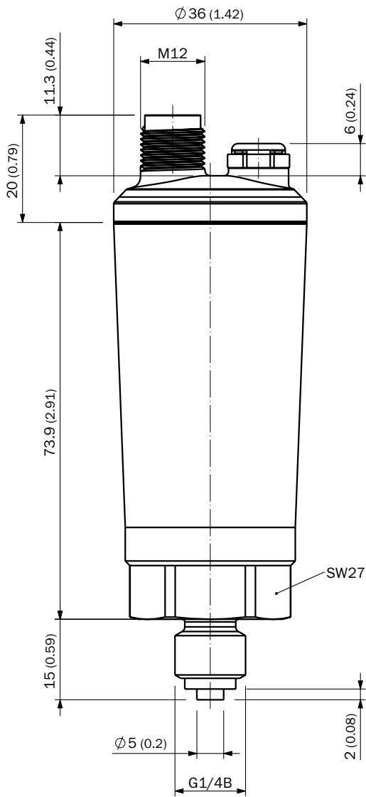
Размеры, мм
