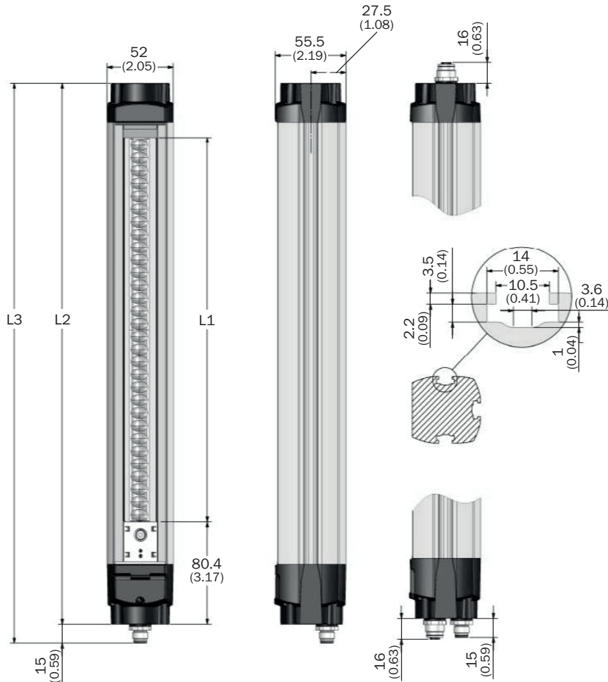
Размеры, мм
