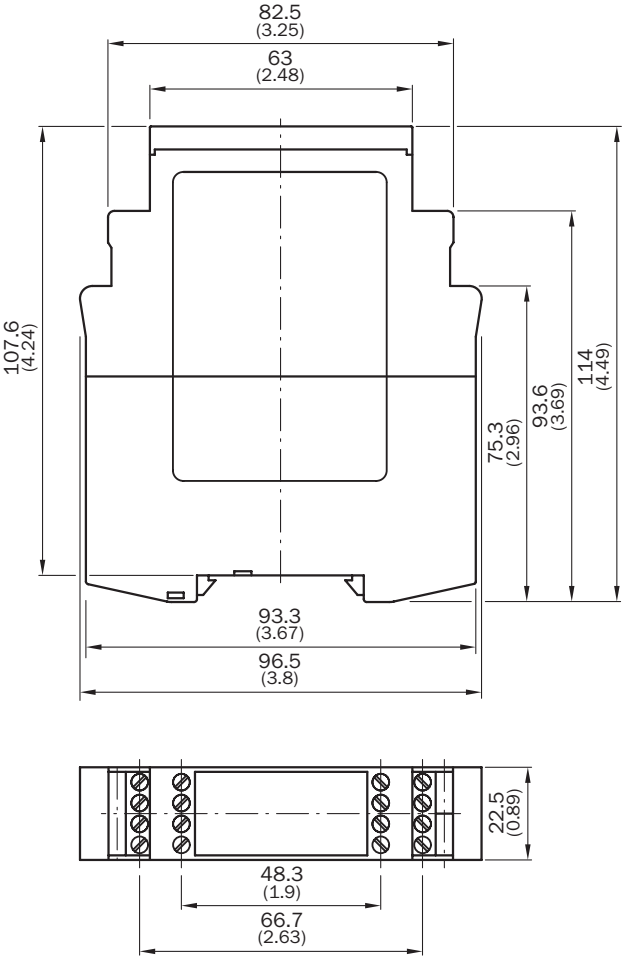
寸法 [mm]
