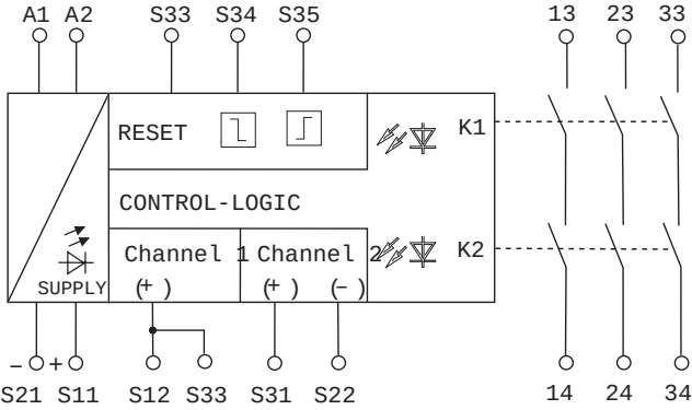
配線図
