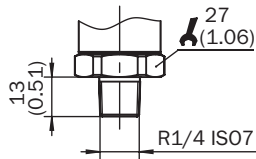
Размеры, мм
