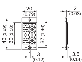
Размеры, мм
