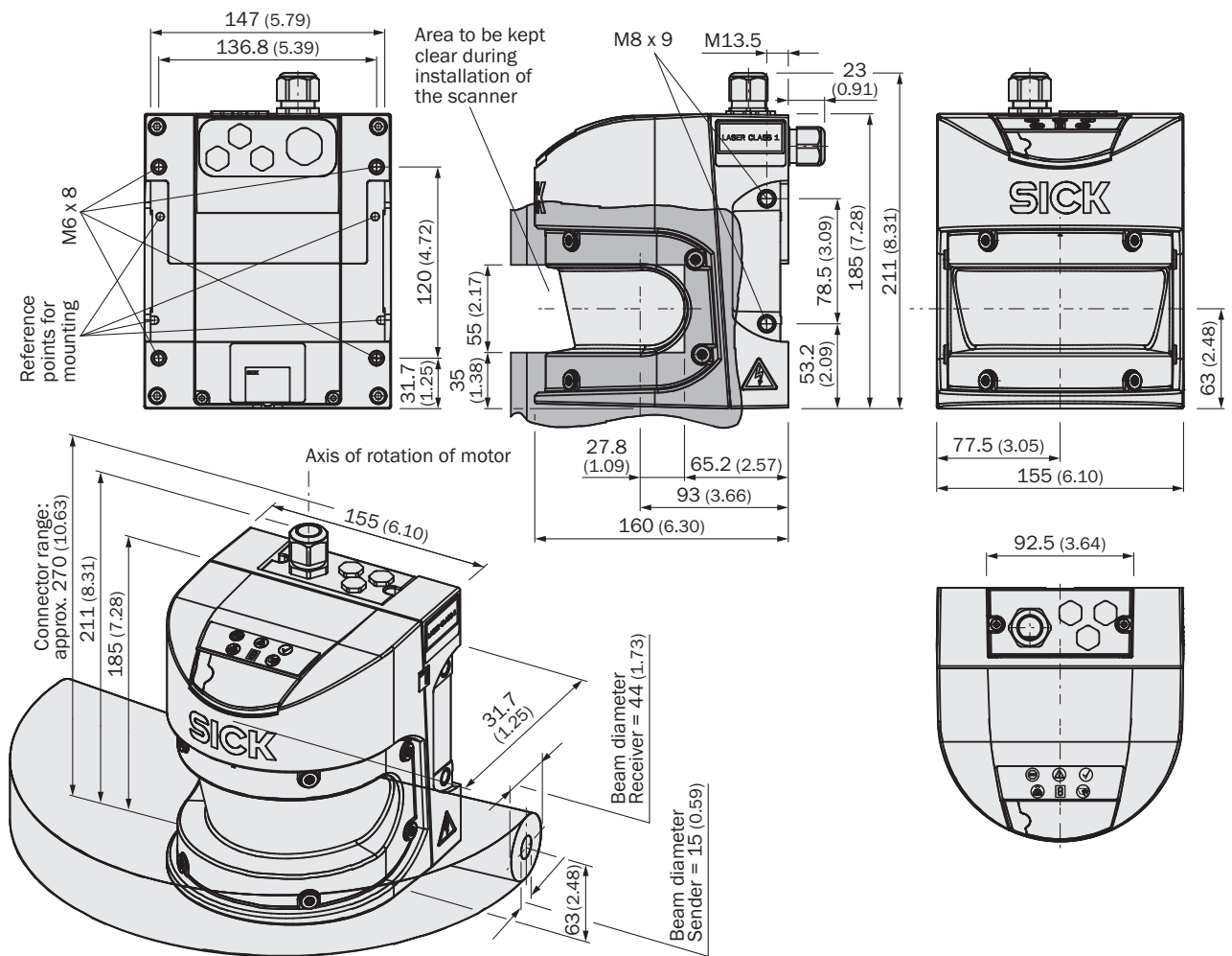
Размеры, мм
