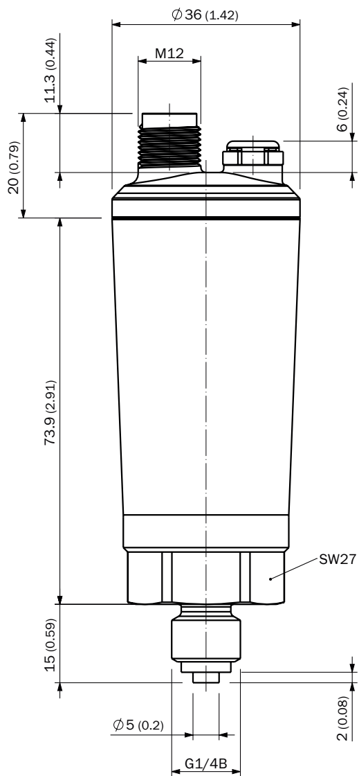
Размеры, мм
