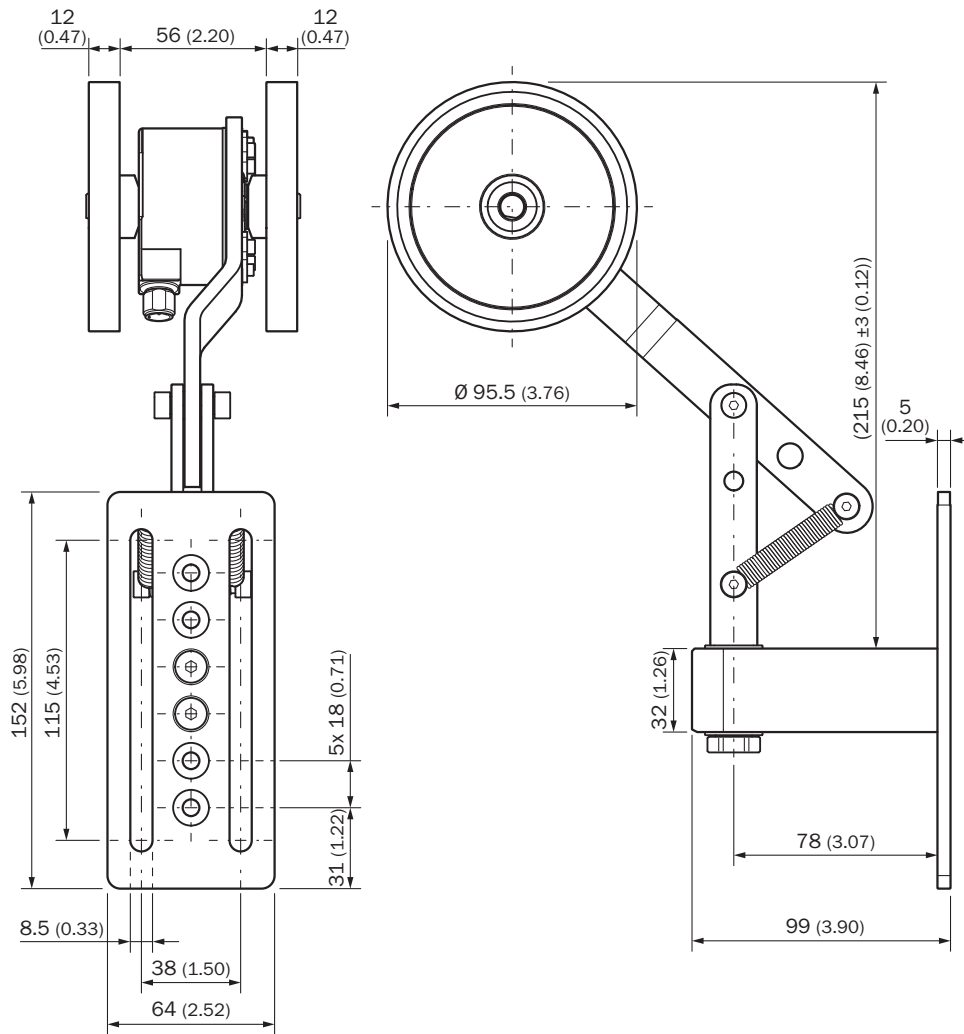
Размеры, мм
