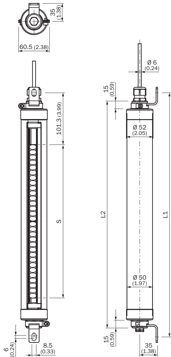
Размеры, мм изображение передатчика (приемник — в зеркальном отображении)
