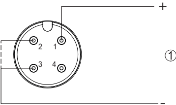
① Источник напряжения и сигнальный выход
