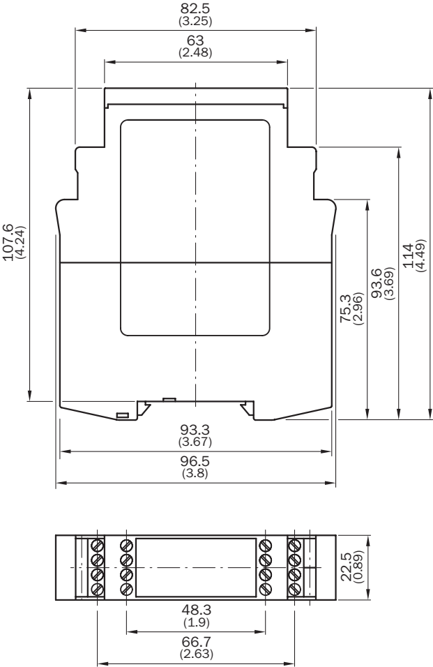
寸法 [mm]
