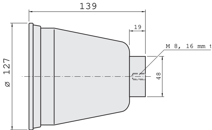
Размеры, мм
