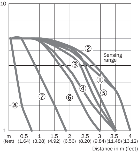
特性曲線 WL11G-2
