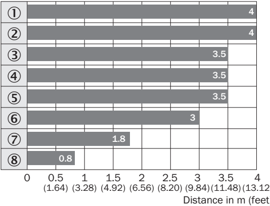
檢測範圍示意圖 WL11G-2
