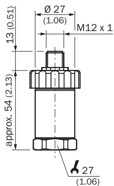
Размеры, мм
