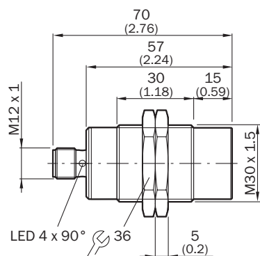
Размеры, мм
