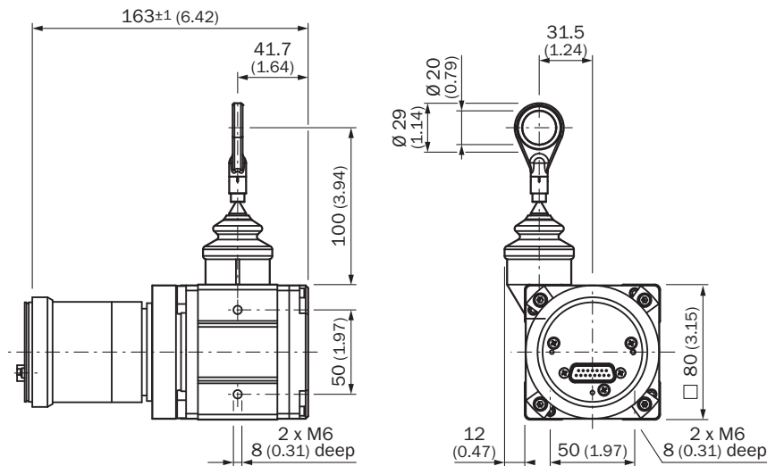
Размеры, мм
