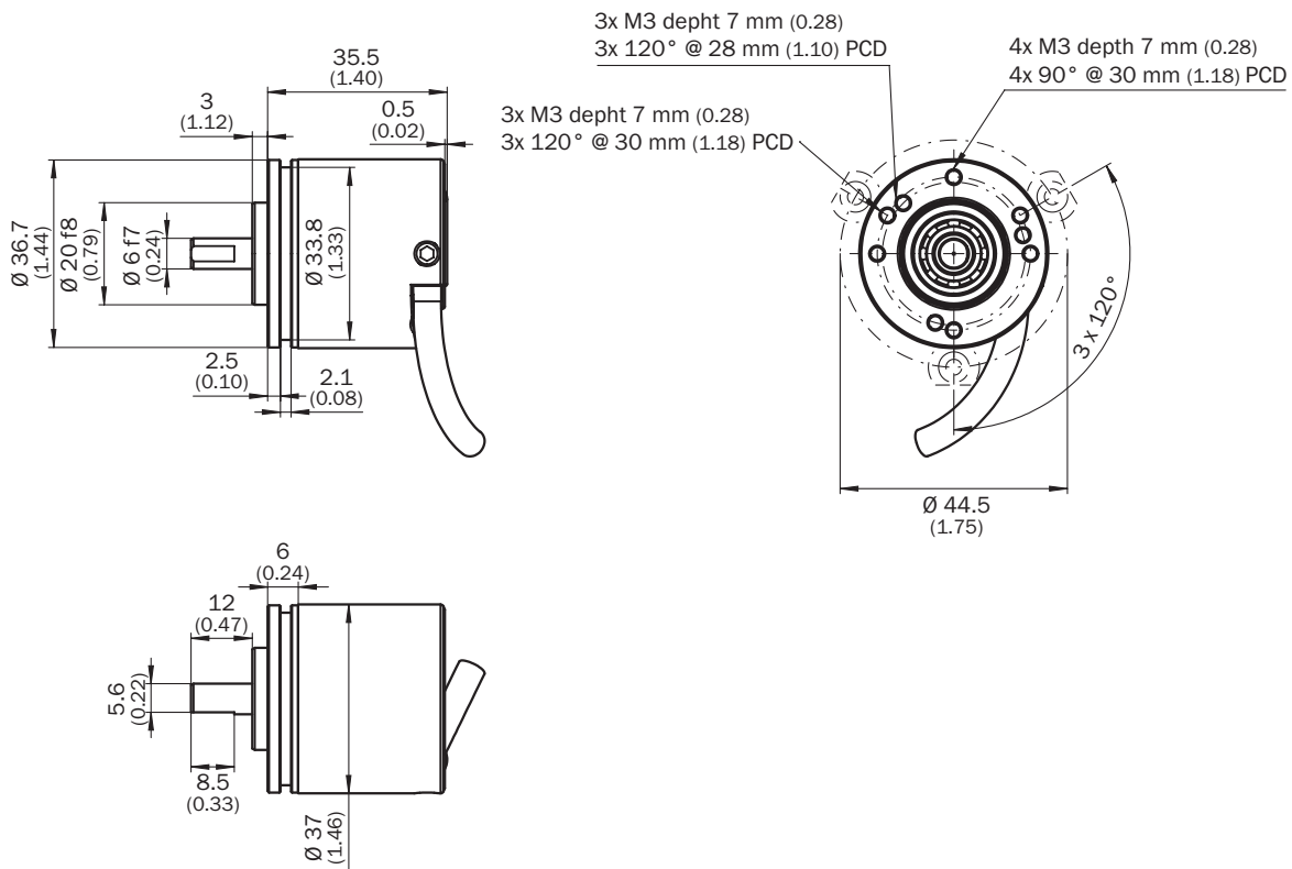
Габаритный чертеж Сплошной вал, захватный фланец, вал 6 x 12 мм, схема расположения отверстий фланца – тип 0
