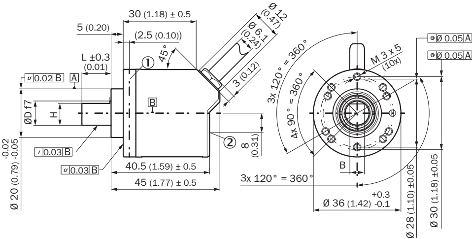
尺寸圖 實心軸，夾緊法蘭，電纜線
