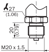
Размеры, мм
