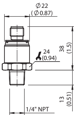
Размеры, мм
