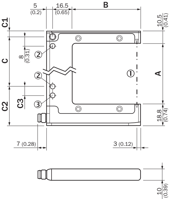
尺寸圖 WFE-XXXXXXX3XX
