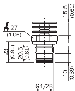
Размеры, мм
