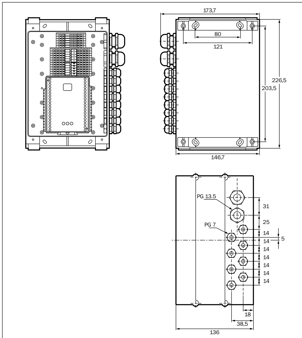
Размеры, мм
