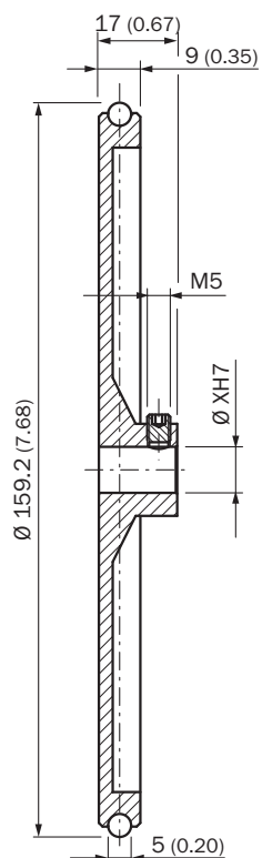
Размеры, мм
