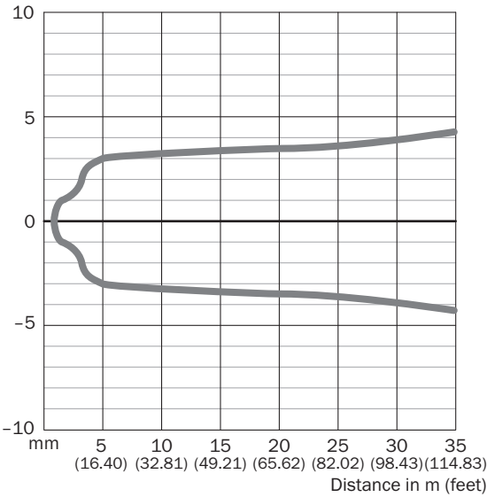
檢測範圍示意圖 VL18 L
