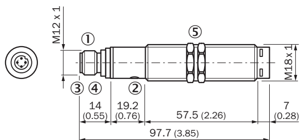
尺寸圖 軸向
