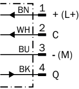
連接示意圖 CD-099
