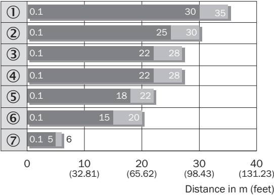
檢測範圍示意圖 VL18 L
