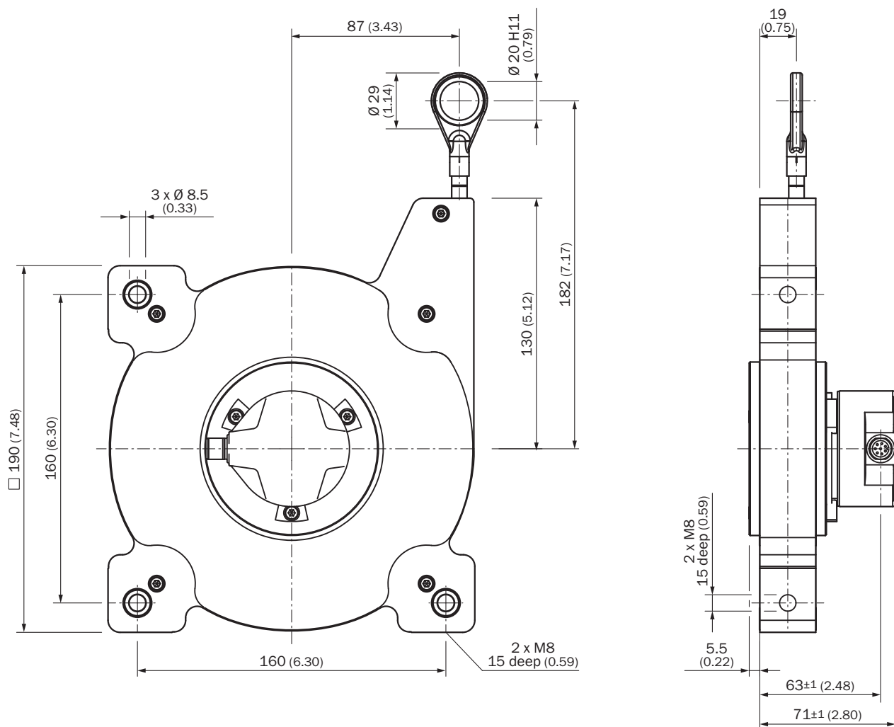
Размеры, мм
